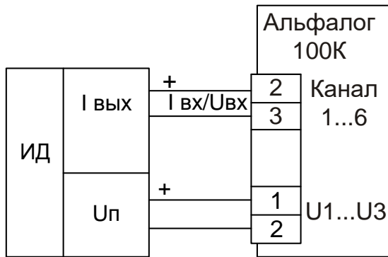
Рисунок 9 – Подключение активных датчиков с унифицированными выходными сигналами тока или напряжения и имеющими раздельные цепи питания
