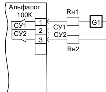
Рисунок 11 – Подключение нагрузки к релейному выходу
