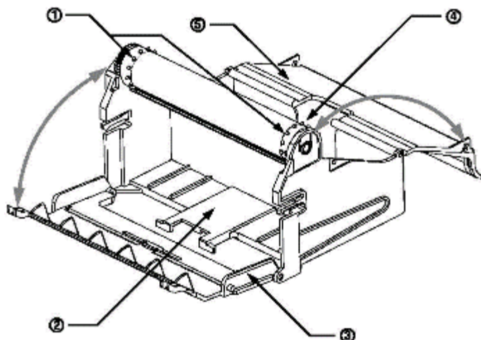
Рисунок 6 – Кассета с бумагой
